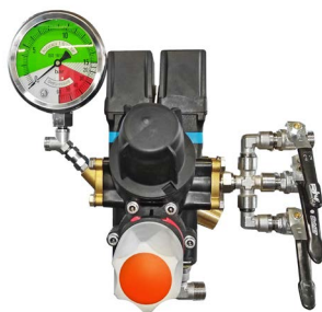
Comando elettrico a 2 vie reg. pressione manuale
