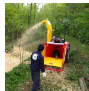
Cippatore CPT130 al lavoro
